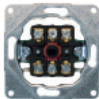
Jalousieschalter / -taster 10 A, 250 V~, 2-polig , Schaltknebel-Ausführung, wahlweise beidseitige Tast- oder Tast-/Rast-Funktion mit PE-Klemme als Tast-/Rast-Version vormontiert
