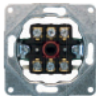
Jalousieschalter / -taster 10 A, 250 V~, 2-polig , Schloss-Ausführung, wahlweise beidseitige Tast- oder Tast-/Rast-Funktion mit PE-Klemme als Tast-/Rast-Version vormontiert
