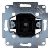
Kreuzschalter 10 A, 250 V~, mit schraublosem Steckanschluss
