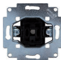
Ausschalter 10 A, 250 V~, 2-polig, mit schraublosem Steckanschluss, Beleuchtungseinsatz nachrüstbar
