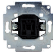
Kontroll-Ausschalter, 2-polig 10 A, 250 V~, inkl. Beleuchtungseinsatz, mit schraublosem Steckanschluss
